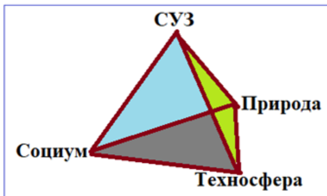
Рис. 1. Система Земля.
